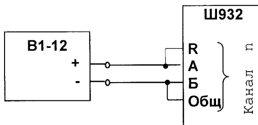
Рисунок Б.1 - Схема для поверки каналов тока Ш932.1, Ш932.2
