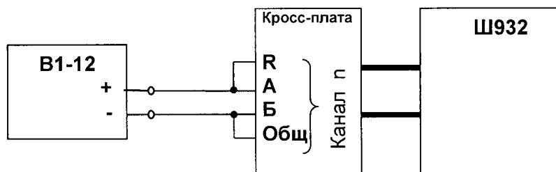
Рисунок Б.4 - Схема для проверки каналов тока Ш932.7, Ш932.9
