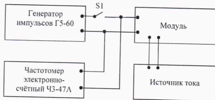
Рисунок 3 - Схема соединений
