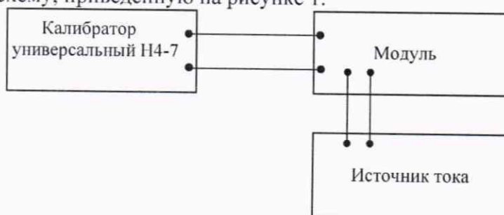
Рисунок 1 - Схема соединений
