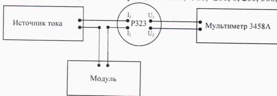
Рисунок 2 - Схема соединений
