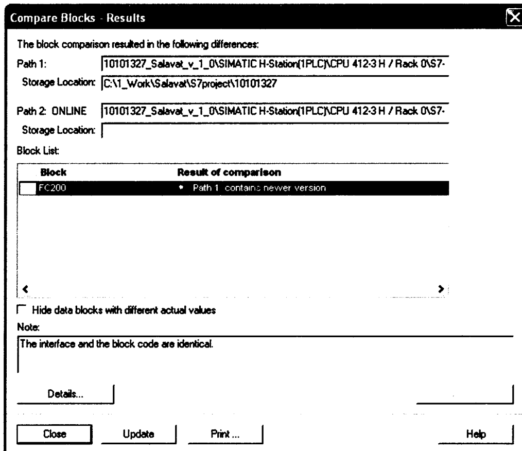
Рисунок 4 – Окно результатов сравнения блока
