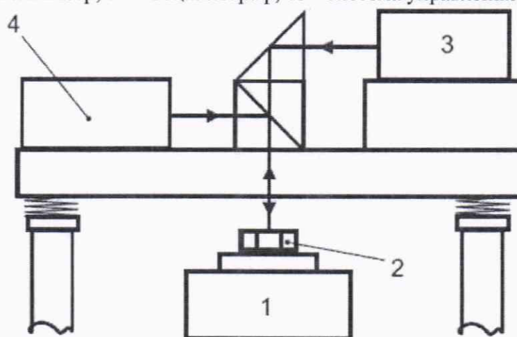
Рис. 3 - Пример схемы совмещения измерительных лучей эталонного лазерного интерферометра из состава ВЭТ (ГЭТ) иверяемого виброметра
