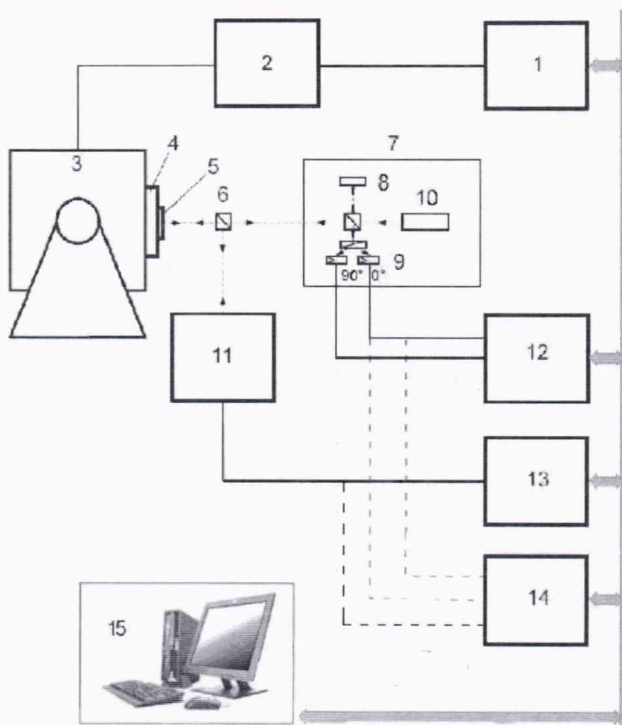
Рис. 2 - Пример установки для поверки лазерных виброметров VibroFlex с помощью ВЭТ (ГЭТ) единиц длины, скорости и ускорения при колебательном движении твердого тела
