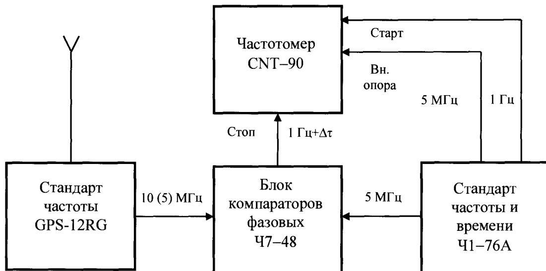
Рисунок 4 – Проверка в режиме синхронизации по сигналам ГНСС относительной погрешности измеренного значения стандарта частоты; нестабильности (СКО и СКДО) измеренного значения стандарта частоты 10 МГц или 5 МГц прибора за 1 с; 10 с; 100 с; 1 сутки
