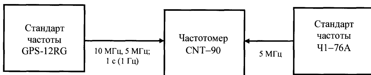
Рисунок 1 – Определение значений частот выходных синусоидальных сигналов 10 МГц и 5 МГц, импульсного сигнала с периодом 1 с
