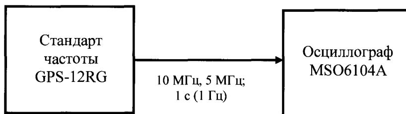
Рисунок 2 – Определение среднего квадратического значения напряжения выходных сигналов 10 МГц (5 МГц).
