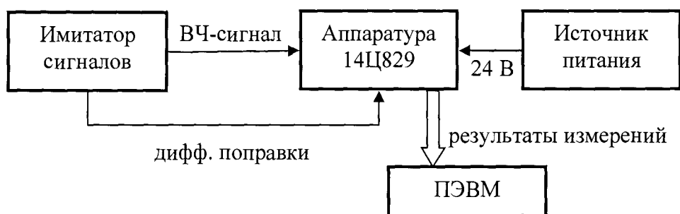
Рисунок 1 - Схема измерений
