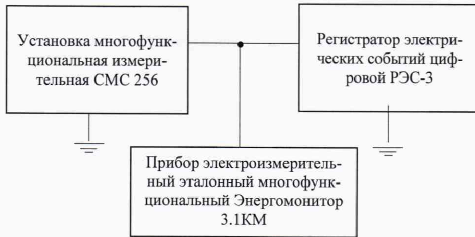
Рисунок 3 – Структурная схема определения погрешностей измерений мощности и коэффициента мощности
