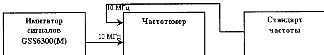
Рисунок 1 – Схема измерений для определения относительной вариации частоты внутреннего опорного генератора за 1 сутки
