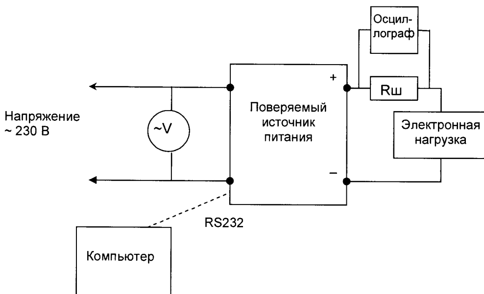
Рис.4 Схема соединений эталонов и поверяемого источника питания
